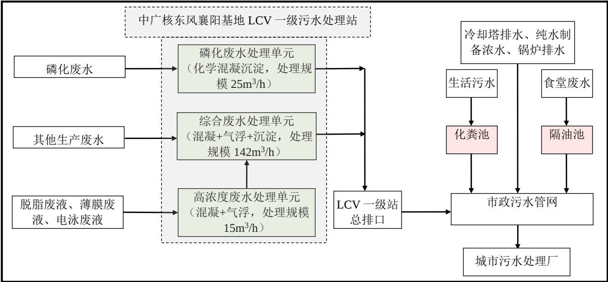
图 6-3-1 项目污水处理总体工艺流程图
