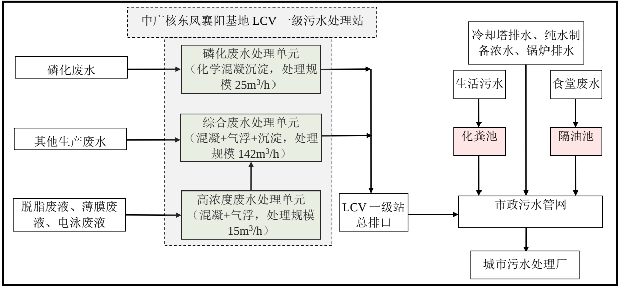
图 3-9-1 东风股份襄阳工厂污水处理总体工艺流程图
