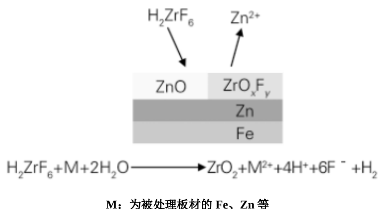
图 4-1-5 锆系薄膜反应机理示意图
