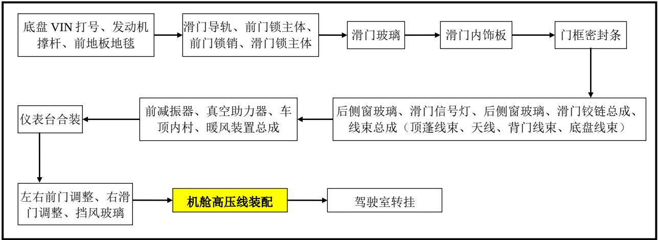
图 4-1-6 内饰装配工艺流程及产污流程图
