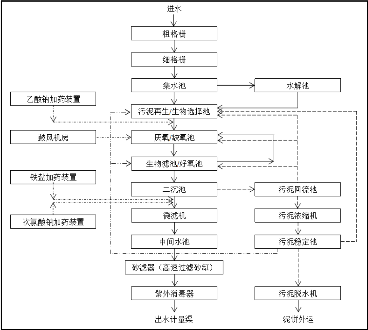
图 6-3-2 中广核环保产业襄阳有限公司高新区污水处理厂工艺流程图 (2) 中广核环保产业襄阳有限公司高新区污水处理厂稳定达标可行性分析
