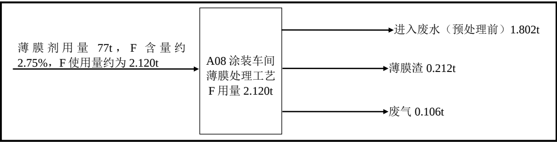
图 4-2-5 项目实施前 A08 涂装车间氟（F）物料平衡图单位：t/a
