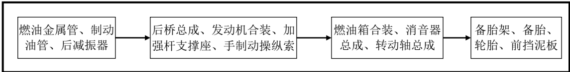
图 2-7-10 底盘装配工艺流程及产污流程图
