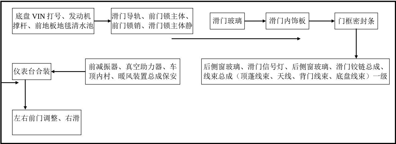
图 2-7-9 内饰装配工艺流程及产污流程图
