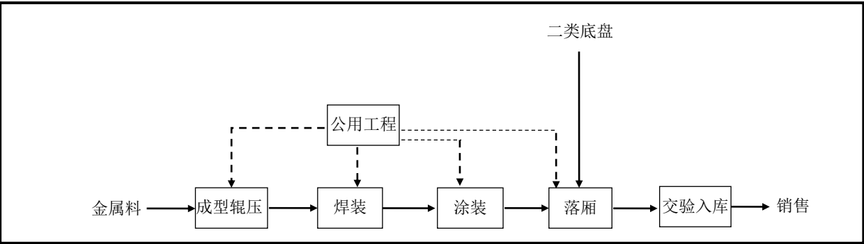
图 2-7-1 车厢生产工艺简图
