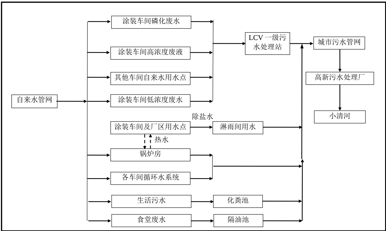
图 3-8-1 项目给排水系统示意图
