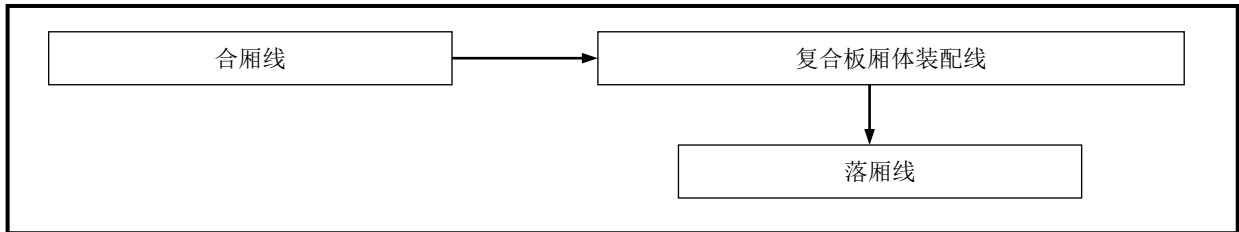
图 2-7-5 车厢落厢车间总体工艺流程示意图
