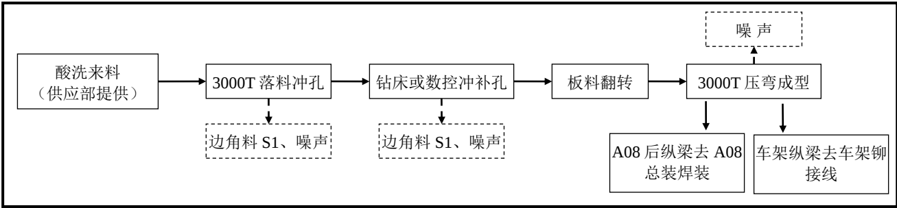
图 2-7-13 纵梁冲压生产工艺及产污流程图
