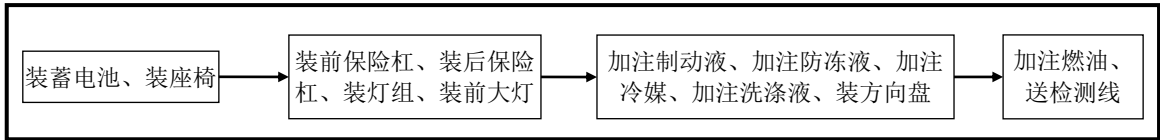
图 2-7-11 最终装配工艺流程及产污流程图
