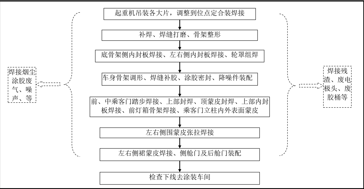
图 2-7-26 焊装车间生产工艺流程及产排污流程图
