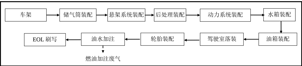
图 2-7-23 北厂区轻卡总装车间车架装配线工艺流程图
