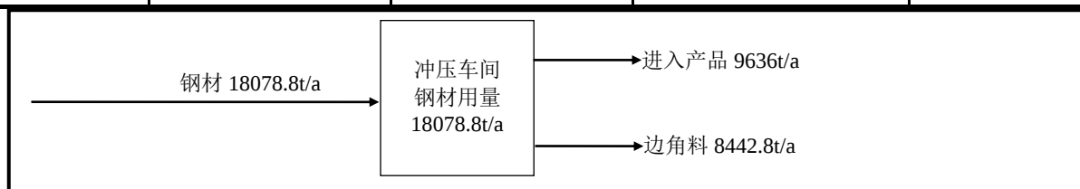
图 4-2-2 项目实施后 A08 冲压车间钢材物料平衡图 单位：t/a
