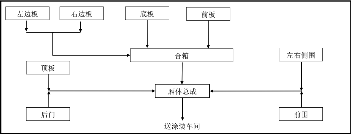
图 2-7-3 车厢焊装线生产工艺及产污环节示意图
