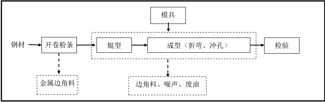
图 2-7-2 成型线生产工艺及产污环节示意图
