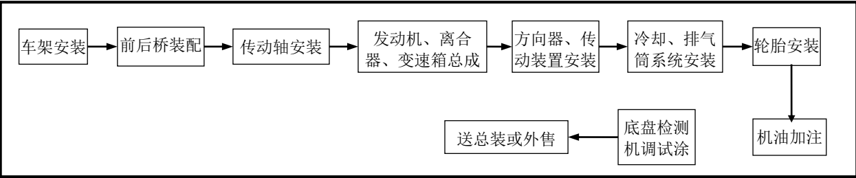
图 2-7-28 底盘装配车间总体工艺流程示意图
