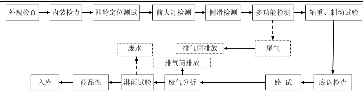
图 2-7-24 北厂区轻卡总装车间内外装/检测线工艺流程图
