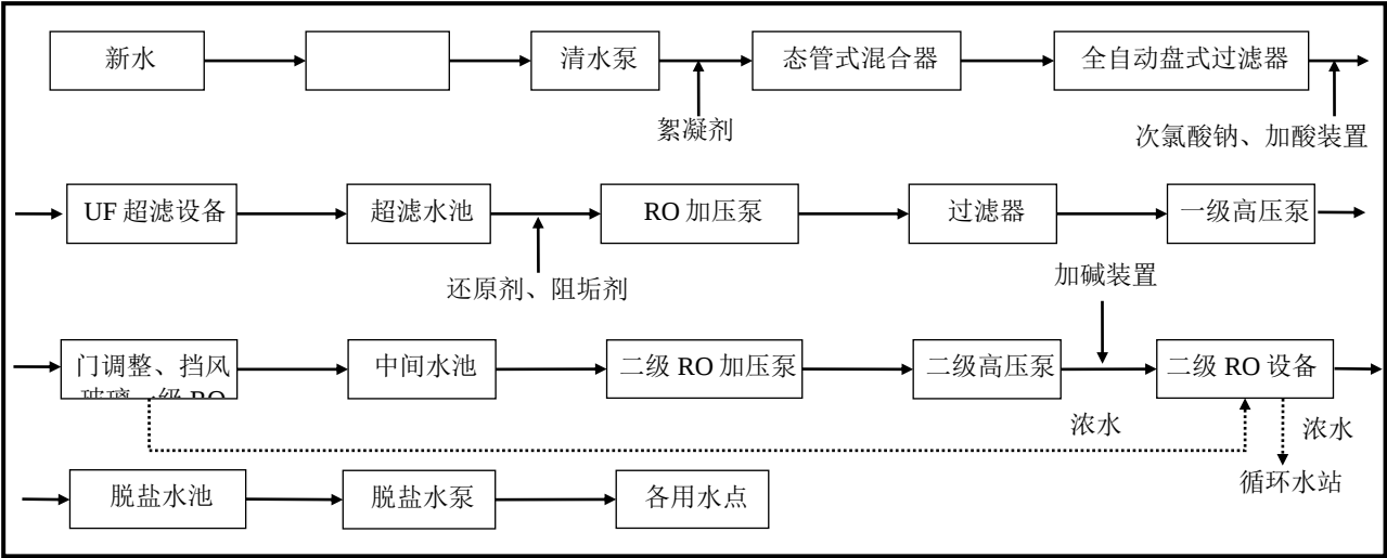
图 2-6-2 现有项目纯水制备工艺流程图
