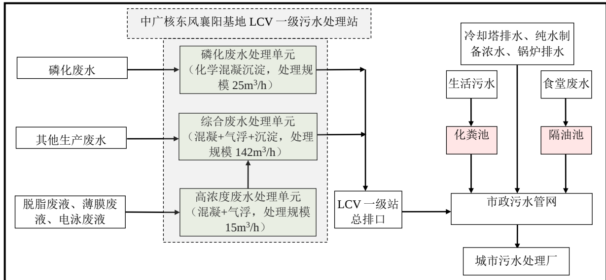
图 4-3-1 项目污水处理总体工艺流程图
