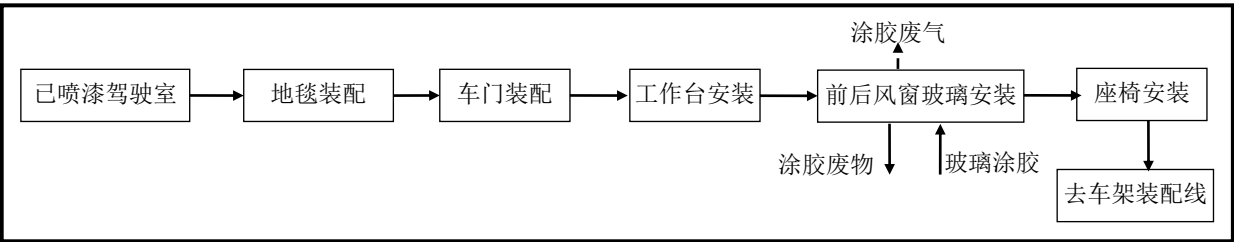
图 2-7-22 北厂区轻卡总装车间内饰线工艺流程图
