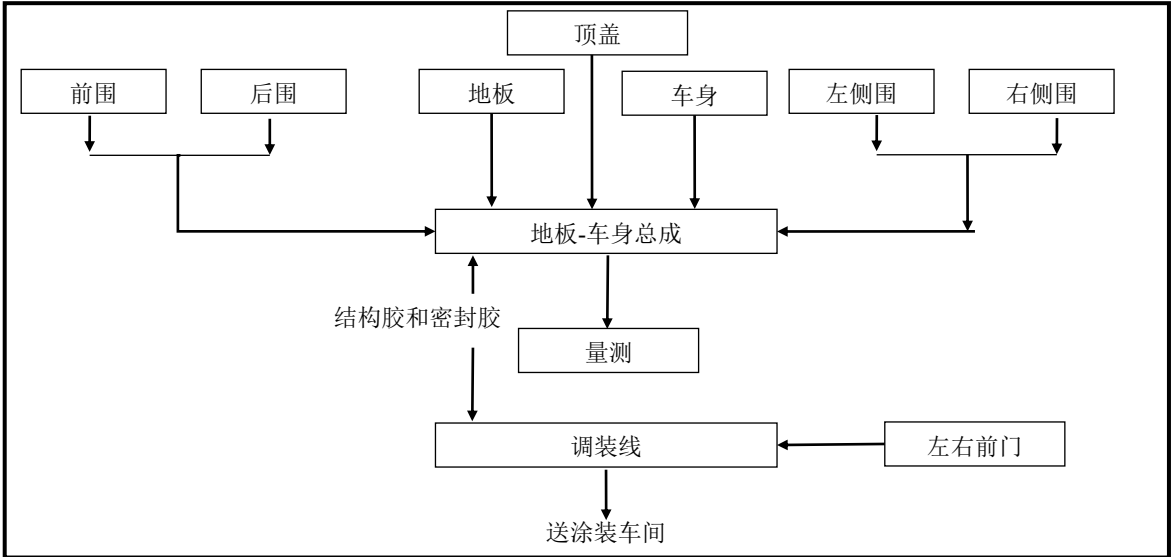
图 2-7-19 轻卡焊装车间总体工艺流程图示意图
